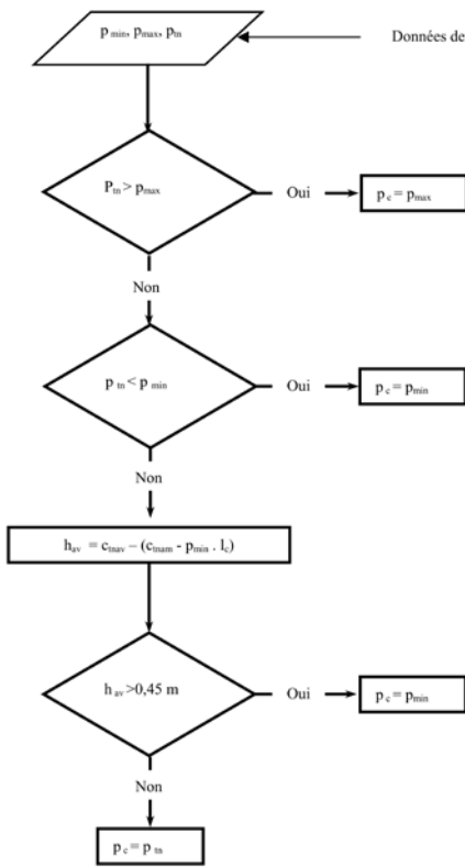
Figure 13.16 : Algorithme de détermination de la pente optimale d'une conduite d'assainissement
