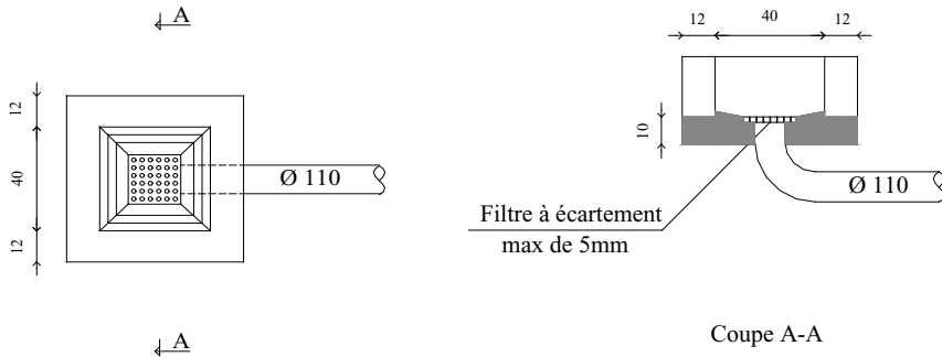
Figure 13.23 : Schéma type de vidoir.
