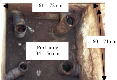
Figure 13.4 : Variation des dimensions des décanteurs
