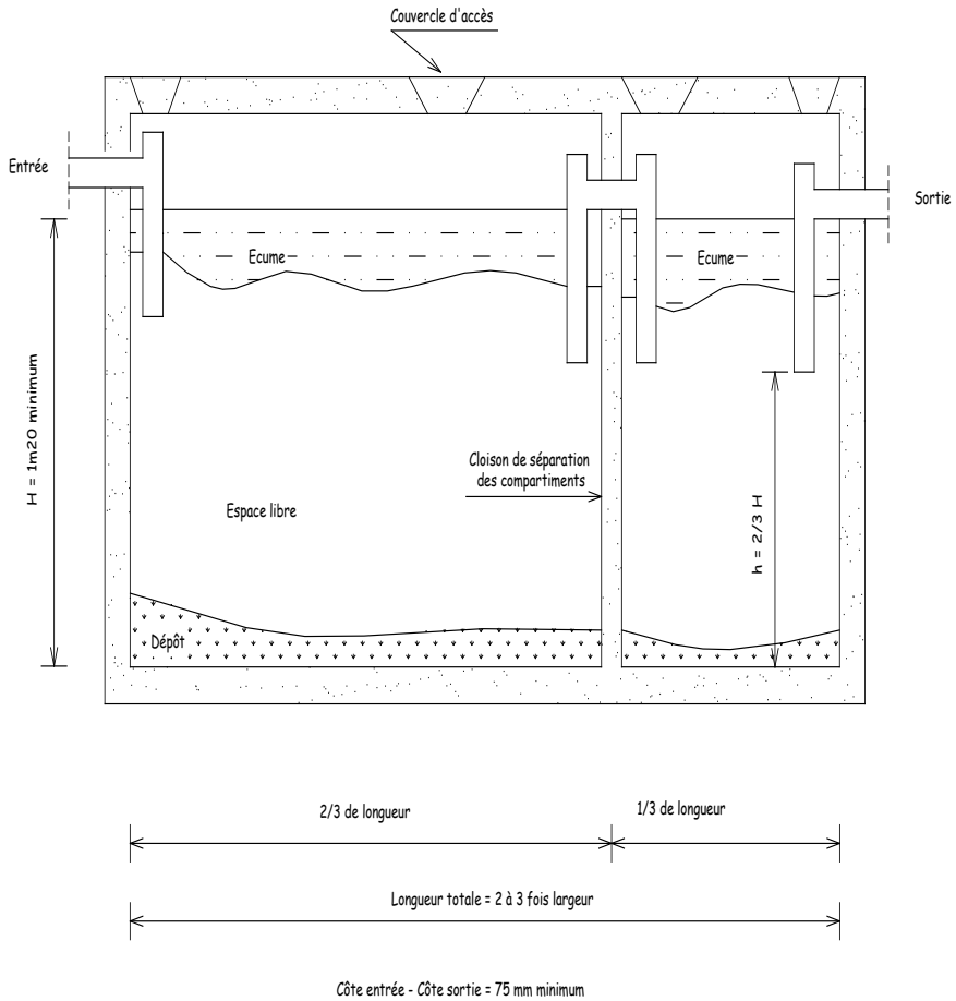
Figure 13.14a : Dispositions constructives des fosses septiques (variante 1).
