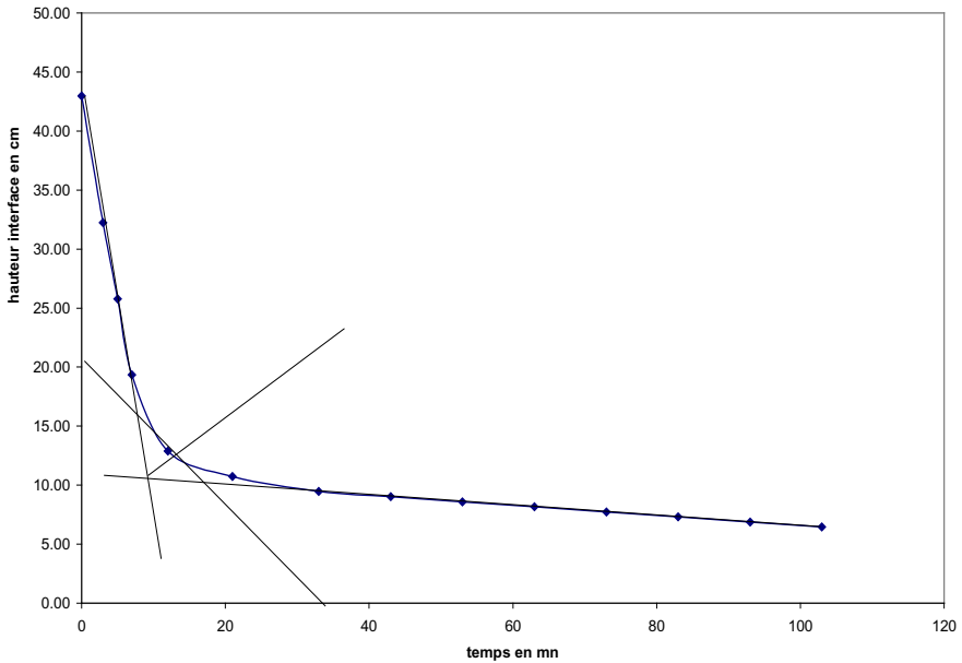
Figure 13.21 : Suivi de la décantation à la station de Castor
