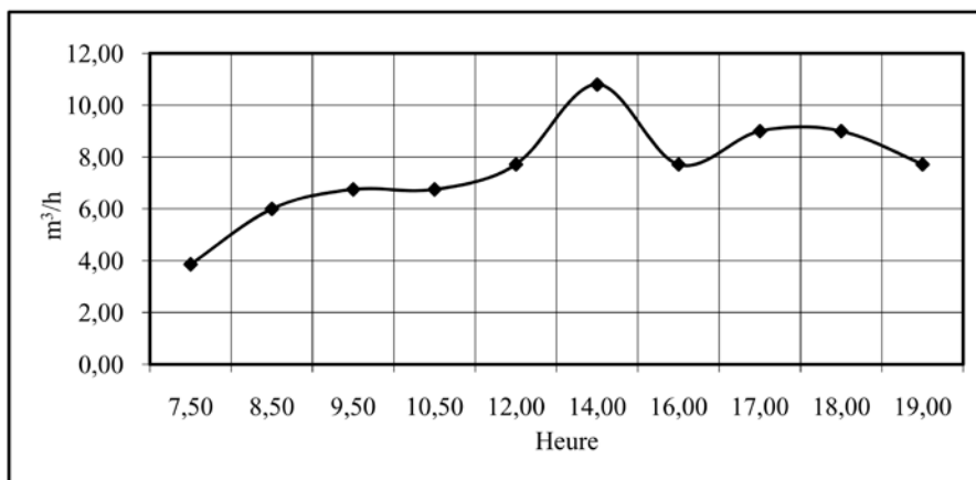
Figure 13.15 : Variation des débits à l'entrée de la station de Castor le 19 février 2002.
