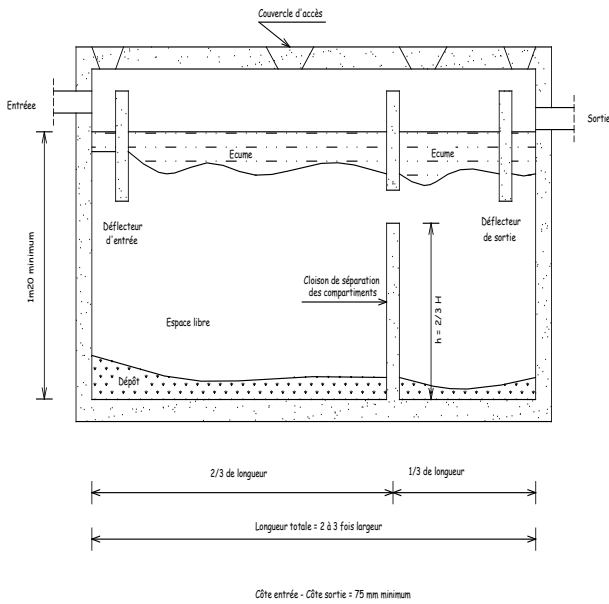
Figure 13.14 b : Dispositions constructives des fosses septiques (variante 2).
