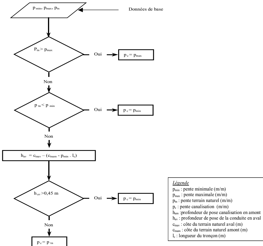
Figure 13.24 : Algorithme de détermination de la pente optimale d'une conduite d'assainissement.
