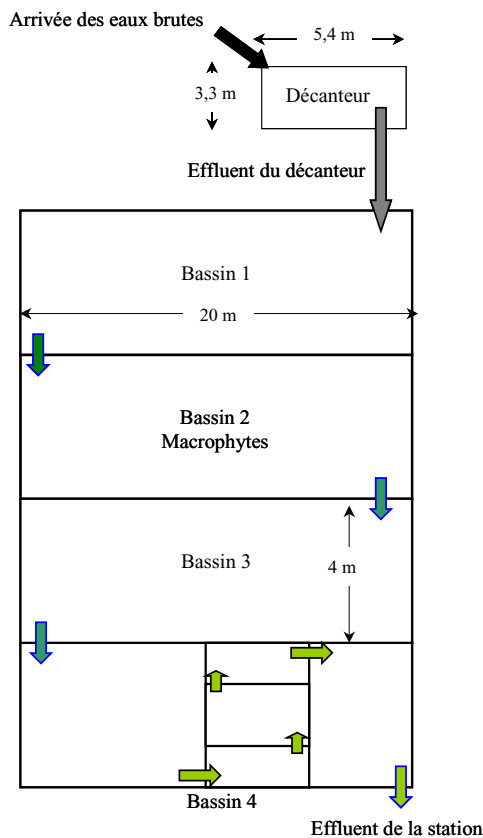
Figure 13.10 : Schéma de la station de Diokoul
