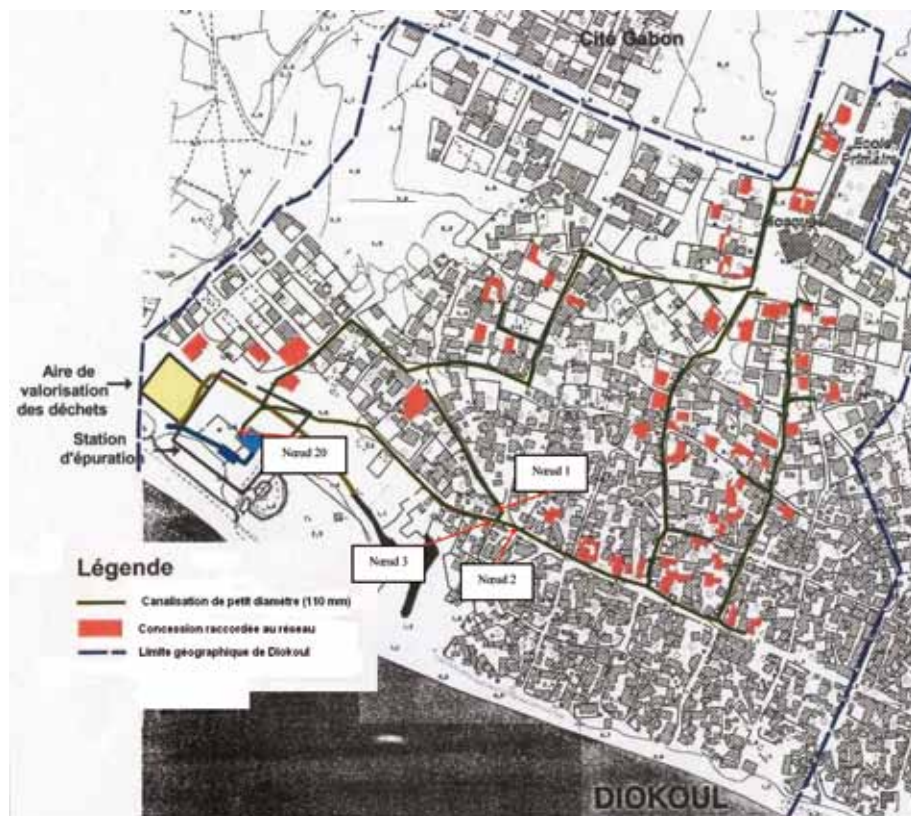
Figure 13.6 : Réseau de Diokoul (Source : ENDA-Rup 2002)
