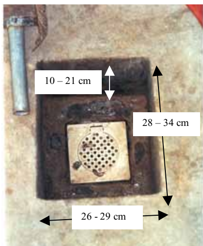
Figure 13.2 : Prototype de viduoir avec les variations de dimensions
